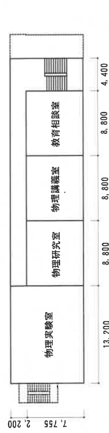
㊦ R4 1号館
